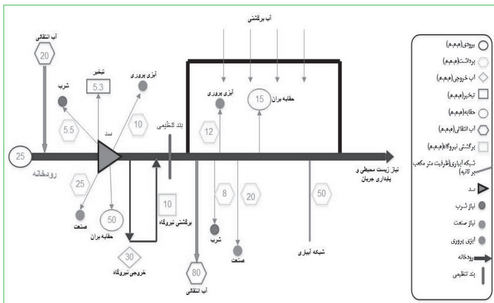
شکل (۲-۱): پیکربندی سیستم طرح سد و نیروگاه‌های برقابی
